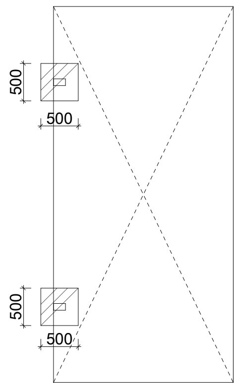
片流れカーポート 2本柱
